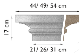
proKERA SANDLINE KAP-II a Ø 20 cm KAP-2 a KAP-II b Ø 25 cm KAP-2 b KAP-II c Ø 30 cm KAP-2 c
