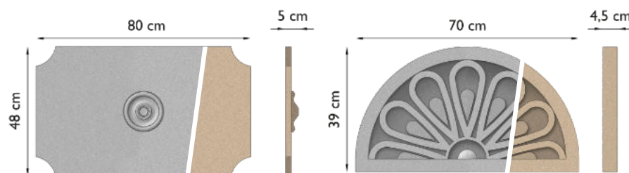
proKERA KERA-Z-1817 inkl. Rosette KERA-RO-1700
