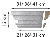
proKERA SANDLINE KAP-IV a Ø 20 cm KAP-4 a KAP-IV b Ø 25 cm KAP-4 b KAP-IV c Ø 30 cm KAP-4 c
