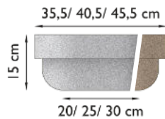
proKERA SANDLINE KAP-I a Ø 20 cm KAP-I a KAP-I b Ø 25 cm KAP-I b KAP-I c Ø 30 cm KAP-I c
