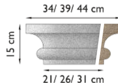
proKERA SANDLINE KAP-V a Ø 20 cm KAP-5 a KAP-V b Ø 25 cm KAP-5 b KAP-V c Ø 30 cm KAP-5 c
