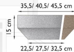
proKERA SANDLINE KAP-III a Ø 20 cm KAP-3 a KAP-III b Ø 25 cm KAP-3 b KAP-III c Ø 30 cm KAP-3 c
