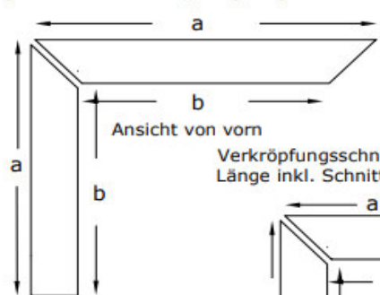
Gehrungsschnitt für Fensterumrahmung Länge inkl. Schnitt = a , Länge zzgl. Schnitt = b
