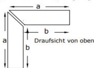
Verkröpfungsschnitt für Hausecken Länge inkl. Schnitt = a , Länge zzgl. Schnitt = b
