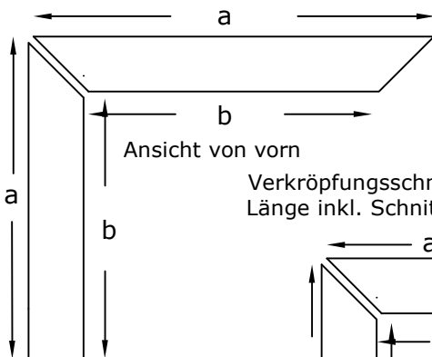
Gehrungsschnitt für Fensterumrahmung Länge inkl. Schnitt = a , Länge zzgl. Schnitt = b
