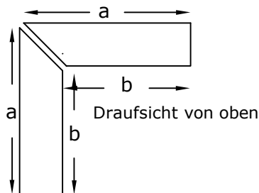
Verkröpfungsschnitt für Hausecken Länge inkl. Schnitt = a , Länge zzgl. Schnitt = b
