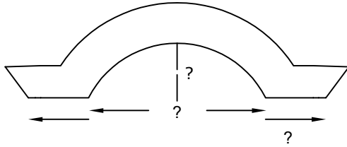
Bogenbekrönung, geteiltes Profil
